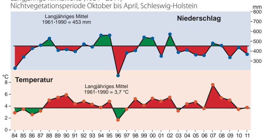
Langjährige Klimawerte (1984 - 2011) Nichtvegetationsperiode Oktober bis April, Schleswig-Holstein
